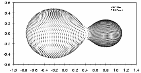
Şekil 3.7. V842 Her yıldızının 0.75 evresindeki geometrik modeli.
