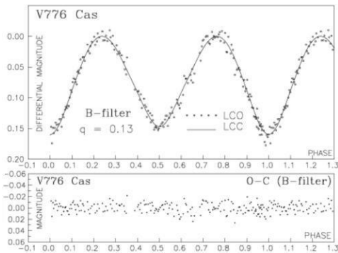
Şekil 3.2. V776 Cas'ın B-bandı gözlemsel ve kuramsal ışık eğrileri ile farkları
