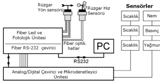
Şekil 1. Donanıma ait blok diyagram
